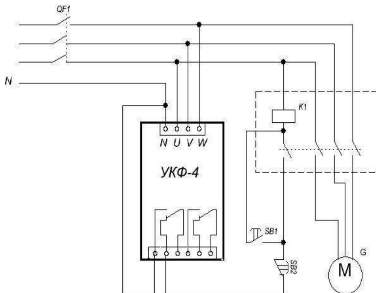
Рисунок 2. Схема подключения
