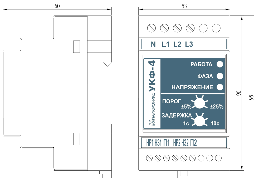
Рисунок 16. Габаритные размеры изделия
